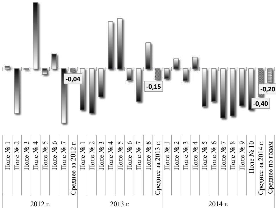
Рис. 2. Коэффициенты корреляции между относительным содержанием хлорофилла в единице площади ассимиляционной поверхности растений озимой пшеницы ( \text{мг}/\text{дм}^2 ) и NDVI
