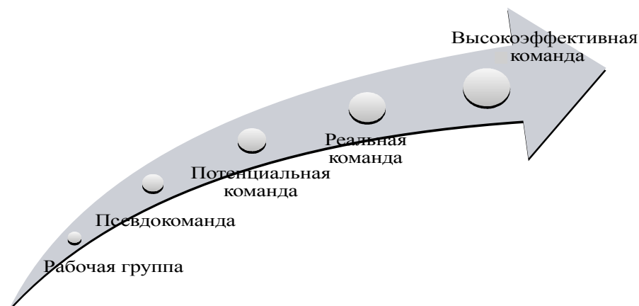
Рис. 2. Процесс командообразования
