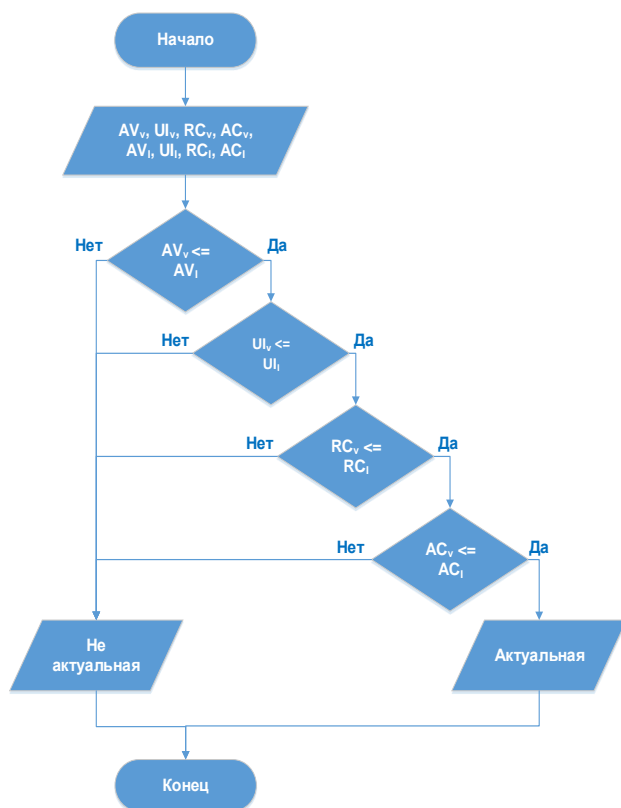
Рис. 3. Блок-схема алгоритма
